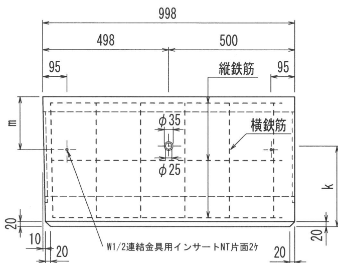
目地部詳細図
