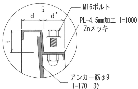
グレーチング受枠詳細図
