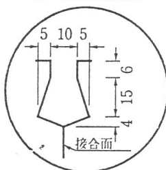
目地部詳細図
