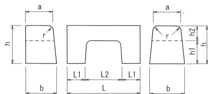
水抜ブロック
