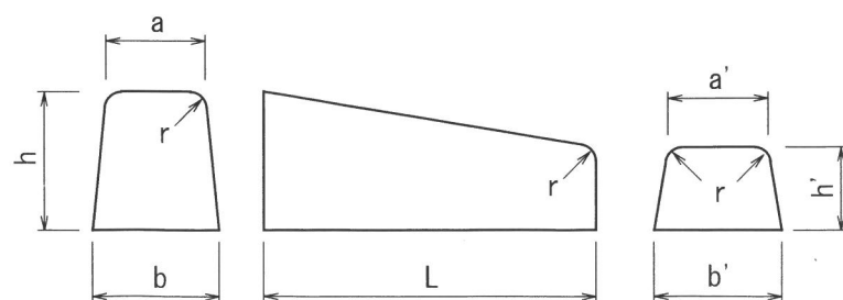
1段乗入ブロック（両面）
