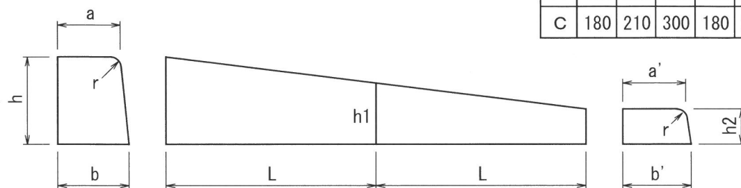
1段乗入ブロック（両面）
