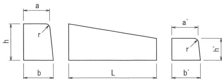
1段乗入ブロック（片面）
