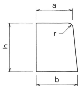
片面歩車道境界ブロック
