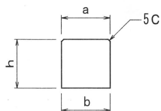
地先境界ブロック
