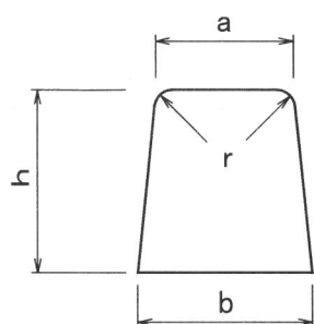
両面歩車道境界ブロック
