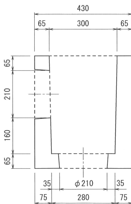
A-A断面図
