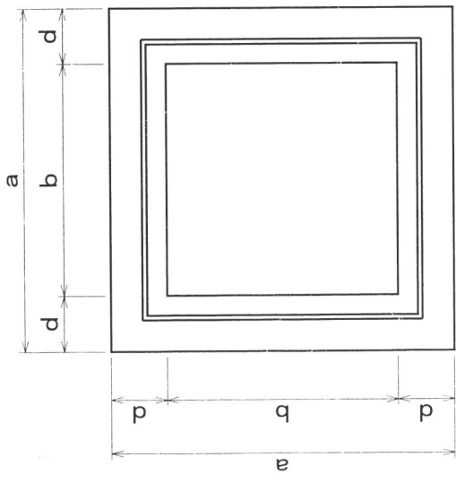
公団樹用受枠
