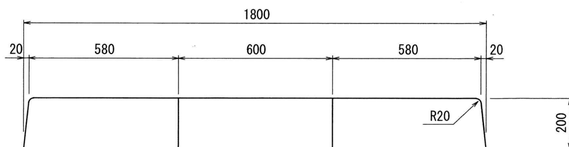
正 面 図
