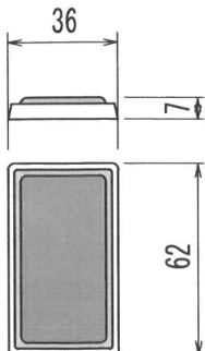
反射鏡
